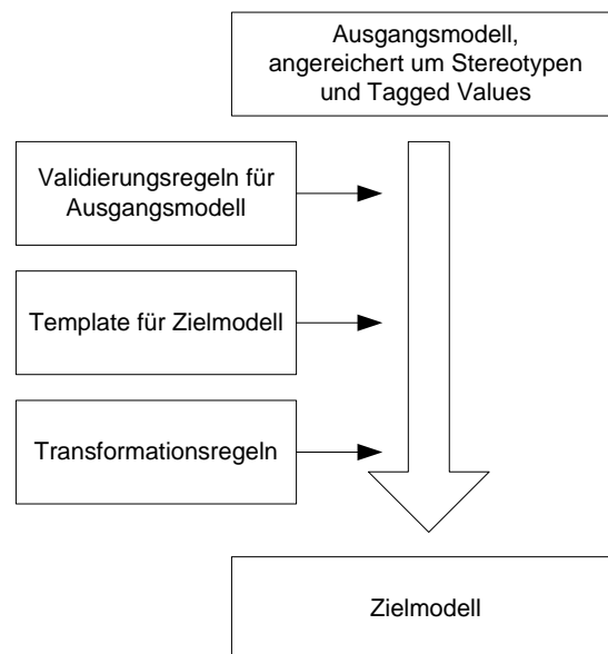
Abbildung 5: Modell-zu-Modell-Transformation
